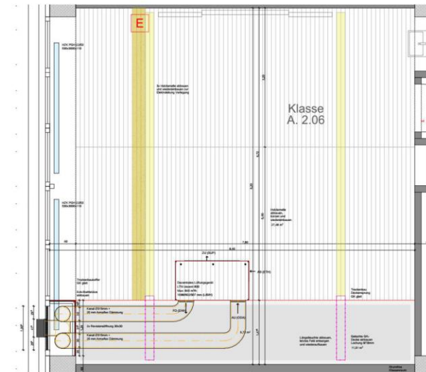
GRUNDRISSE DECKENUNTERSICHT
