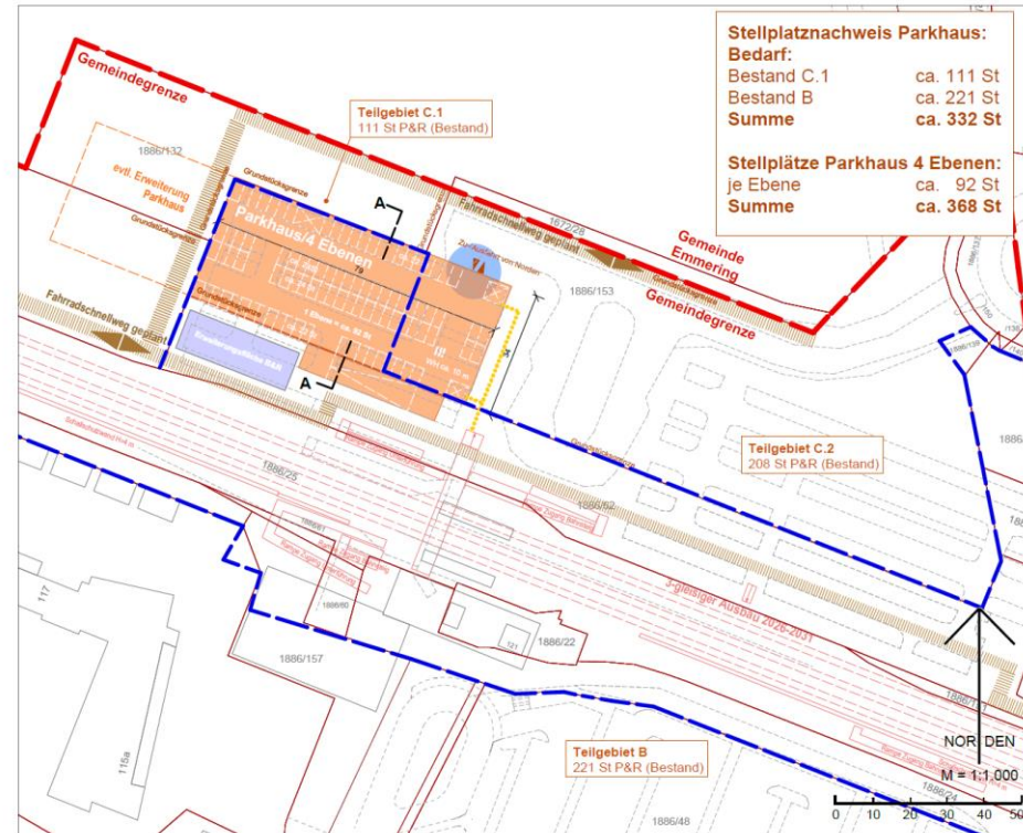
Rahmenplan Ausschnitt Teilbereich C
